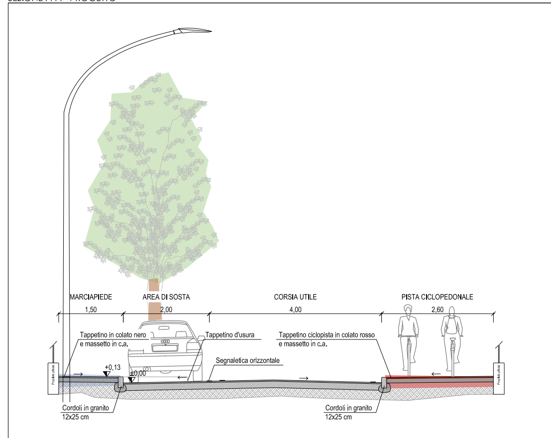
SEZIONE A-A - PROGETTO
