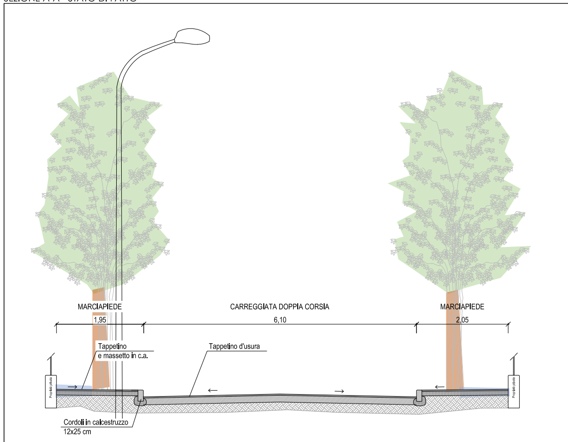
SEZIONE A-A - STATO DI FATTO
